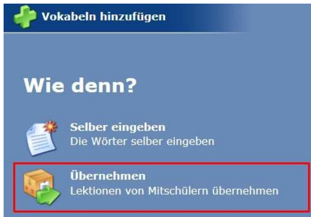
Abb. 10 - Übernehmen auswählen
