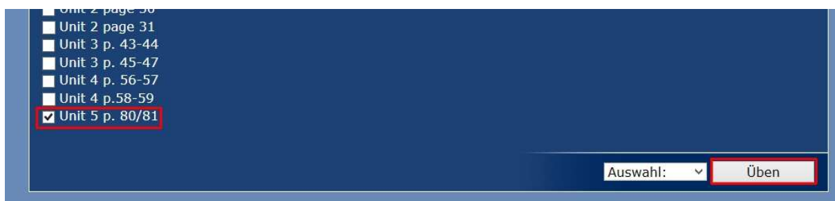
Abb. 2 - Lektion auswählen
