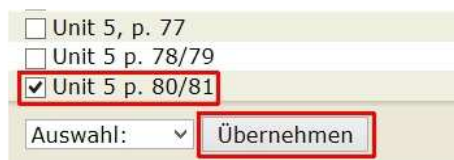
Abb. 12 - Lektion auswählen
